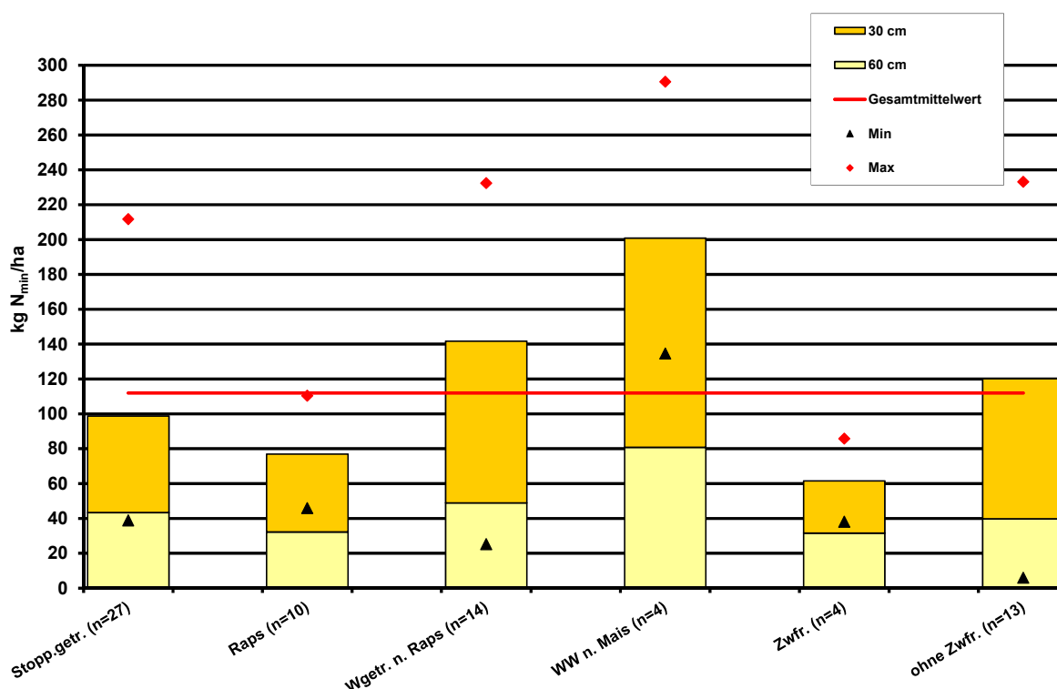
Abbildung 2: Herbst- N_{\min} -Ergebnisse 2018 nach ausgewählten Kulturen im Maßnahmenraum
